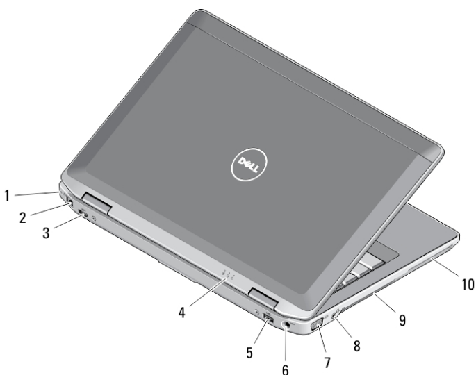
Obrázek 2. Pohled zezadu
